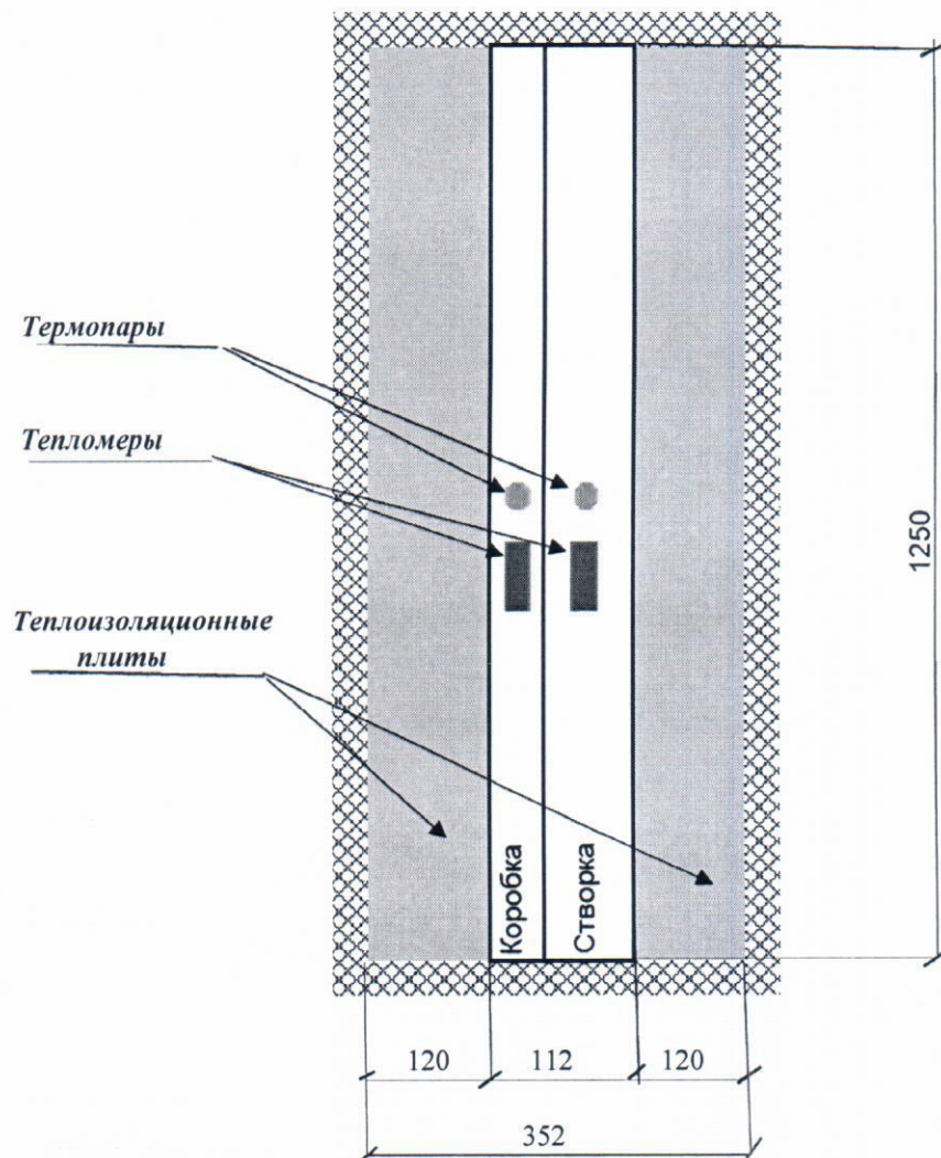
Схема размещения термопар и тепломеров на испытываемом образце комбинации профилей поливинилхлоридных (коробка/створка) т.м. PROPLEX системы HIT
